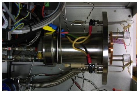
Preconcentration (Medusa)
